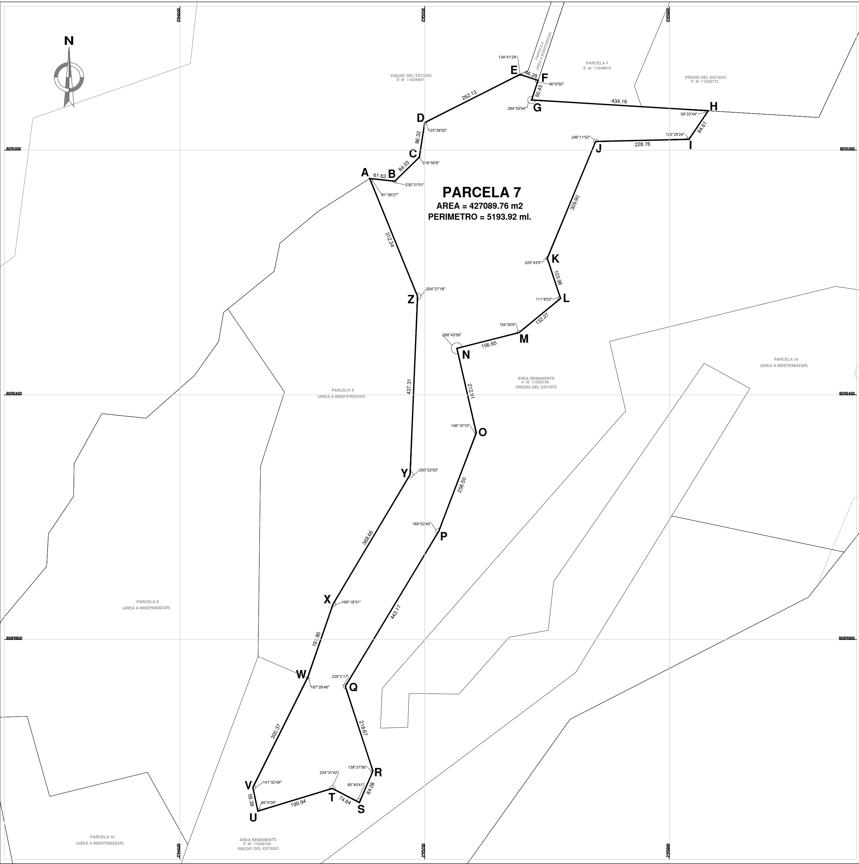
PLANO PERIMÉTRICO POLIGONO GRAFICADO EN PSAD 56 ZONA 19 SUR - ESC. 1/7500
